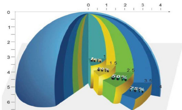
Erfassungsbereich des Bewegungsmelders
