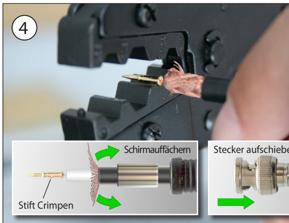
4.) Innenleiterstift Crimpen, Masseschirmauffächern
