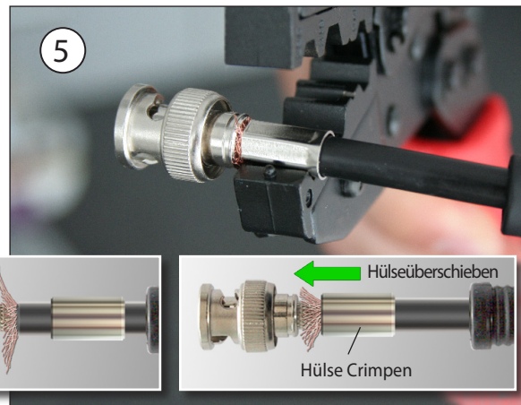
5.) Stecker aufschieben, Massehülse Crimpen
