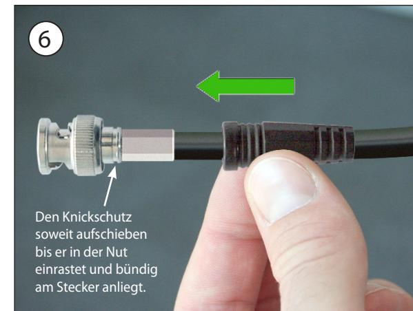
6.) Knickschutz überschieben
