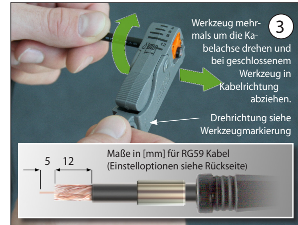
3.) Schirm und Mittelleiter abisolieren
